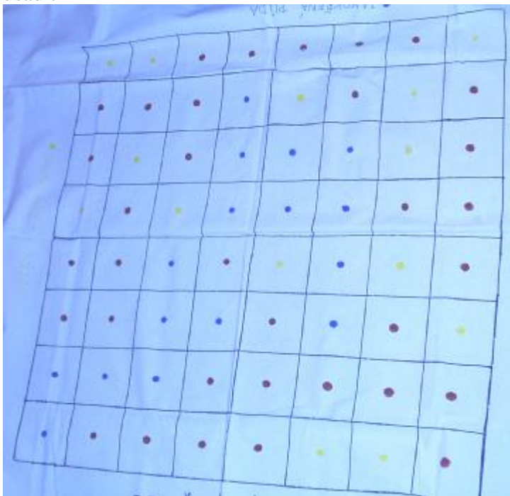
Obr. 1: Hrací pole
